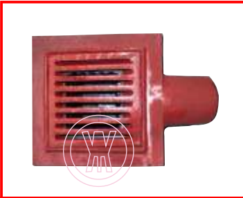
27x27 Q70 Yandan Çıkışlı Pik Süzgeç
