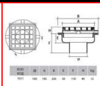
YS 11 Otopark Süzgeci (Sifonlu)
