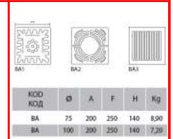
BA Serisi Çatı ve Balkon Süzgeci
