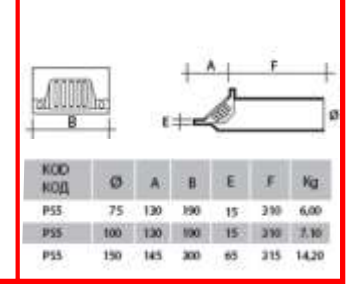
P Serisi Parapet Süzgeci (Yatay Çıkışlı)
