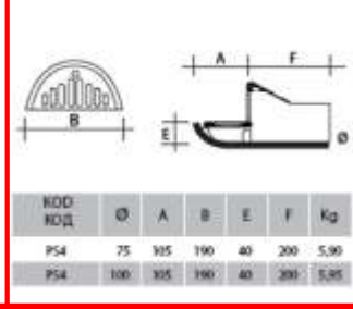
P Serisi Parapet Süzgeci (Yatay Çıkışlı)
