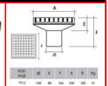
YS 12 Otopark Süzgeci (Sifonsuz)
