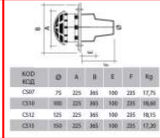
CS Serisi Pik Çatı Süzgeci (Altan)
